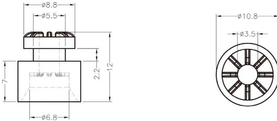
LTGM42 结构图
